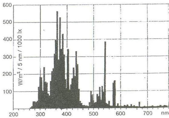
UVA 波長圖
