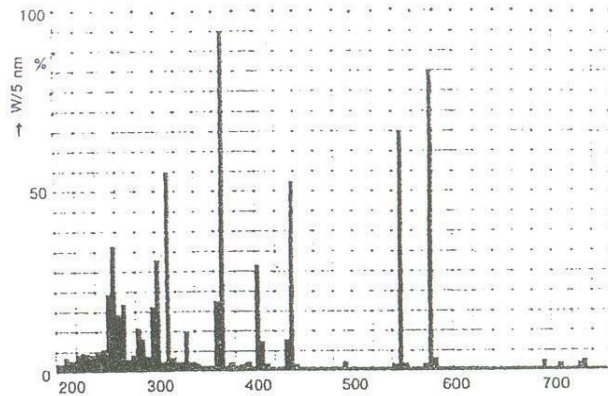
UVC 波長圖
